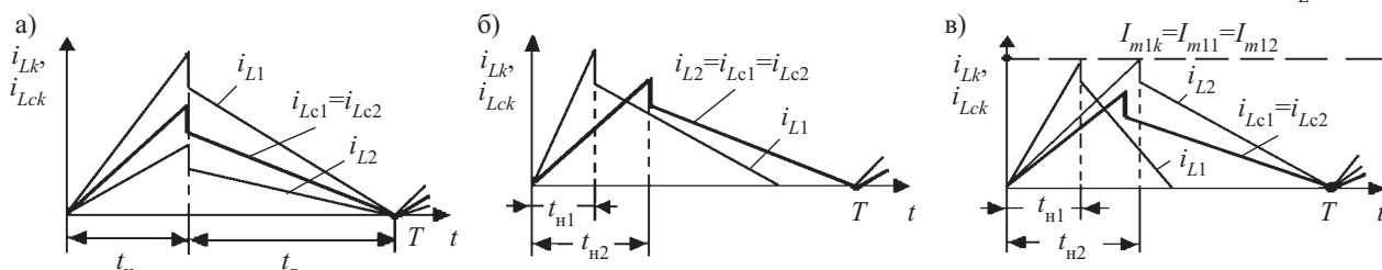
Рис. 4. Временные диаграммы, иллюстрирующие особенности функционирования схем управления CY1 (а), CY2 (б) и CY3 (в) при N=2
