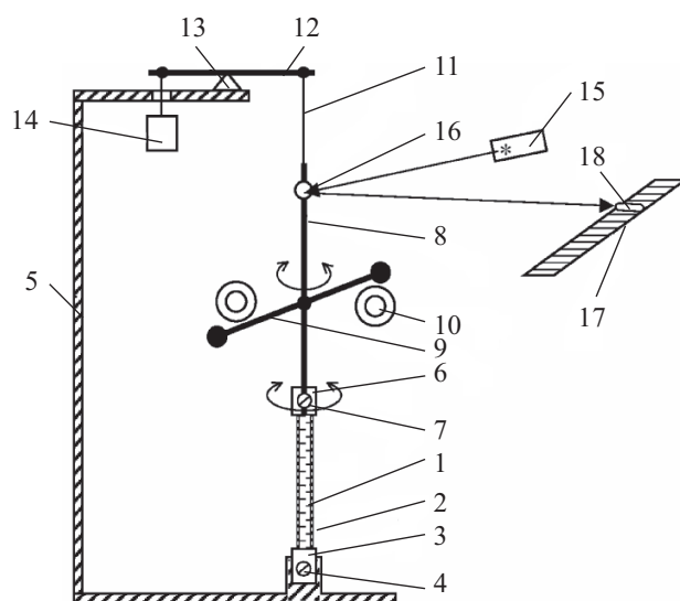
Рис. 1. Схема реализации базового (визуального) способа определения параметров колебаний крутильного маятника: 1 — исследуемая жидкость; 2 — трубка из эластичного материала; 3, 6 — пробка; 4, 7 — зажим; 5 — штатив; 8 — жесткий стержень; 9 — коромысло; 10 — электромагнит; 11 — упругая нить; 12 — рычаг подвесной системы; 13 — опора; 14 — груз натяжения; 15 — источник света (лазер); 16 — зеркало; 17 — шкала; 18 — пятно от луча света на шкале
