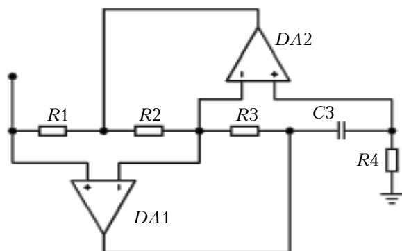
Рис. 2. Схема эквивалентной индуктивности на операционных усилителях
