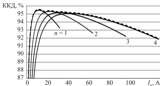
Рис. 7. Залежність ККД багатofазного перетворювача від струму навантаження I_n для різної кількості фаз n
