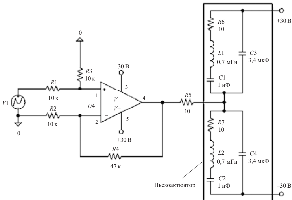
Рис. 5. Электрическая схема усилителя пьезоактуатора изгибного типа
